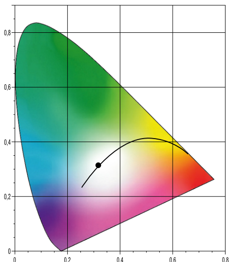
NORMFARBWERTANTEILE X,Y CIE 1931
